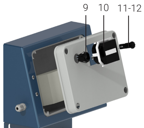
Platine électrique
